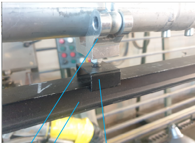
1KB Binario + 1KAS Attacco per sospensione + Aliscat
